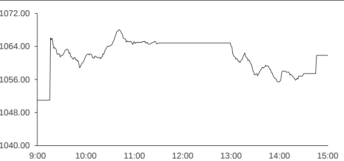
Hình 1 HSX-Index Intraday
