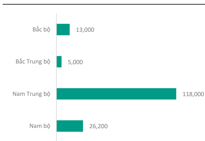
Hình 3: Tiềm năng điện gió ngoài khơi của Việt Nam theo khu vực (MW)
