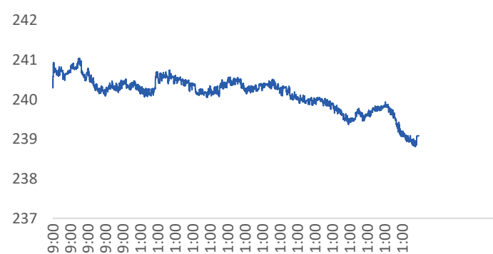
Hình 2 HNX-Index Intraday
